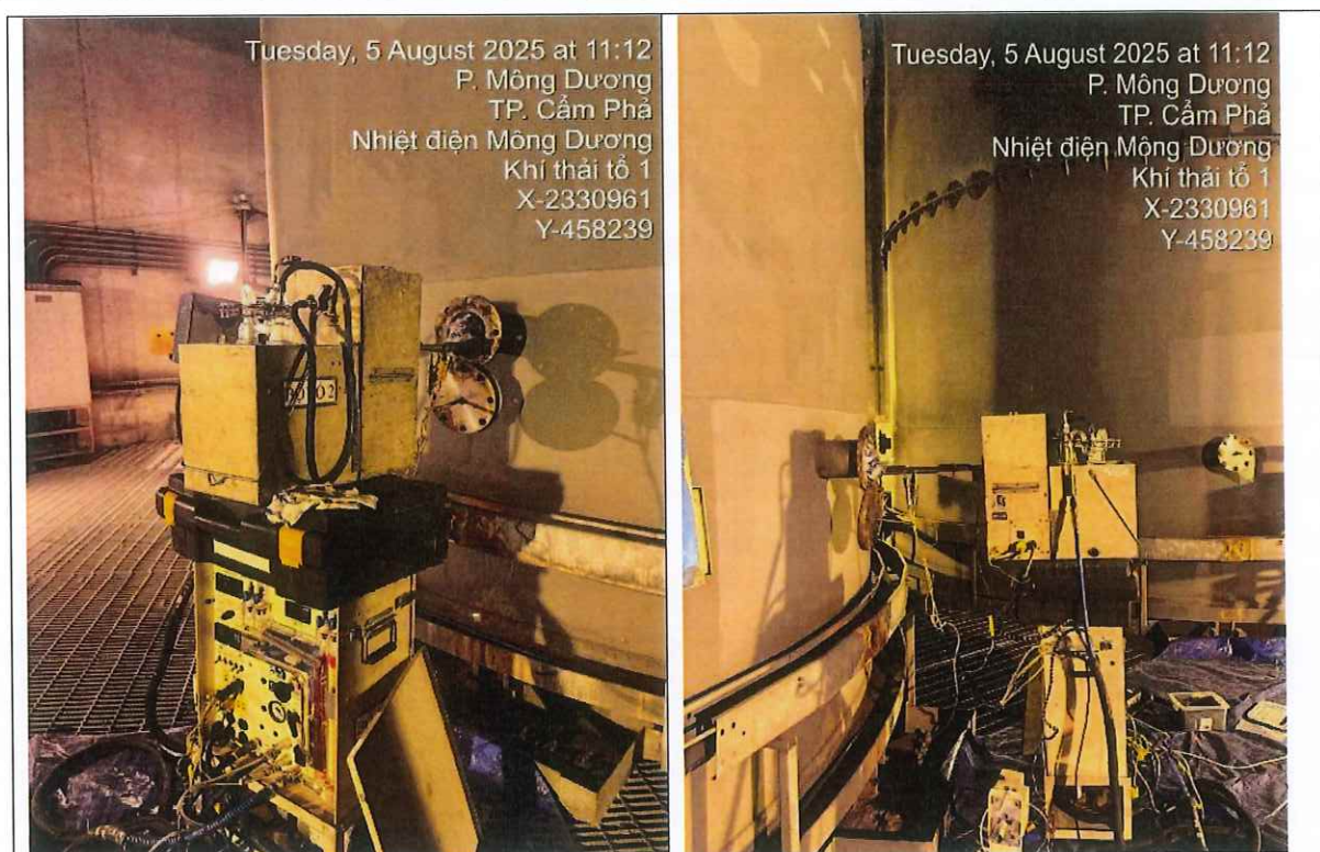
Hình 4.4. Lấy mẫu khí thải trong nhà máy
